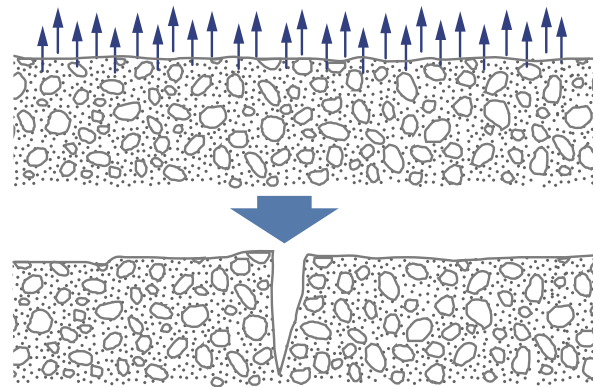
Schrumpfen des plastischen Betons kann durch den Unterdruck, der beim Austrocknen in den mit Flüssigkeit gefüllten Poren entsteht, zu Rissen führen.
